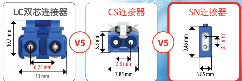
LC, CS, SN 三款连接器尺寸对比
